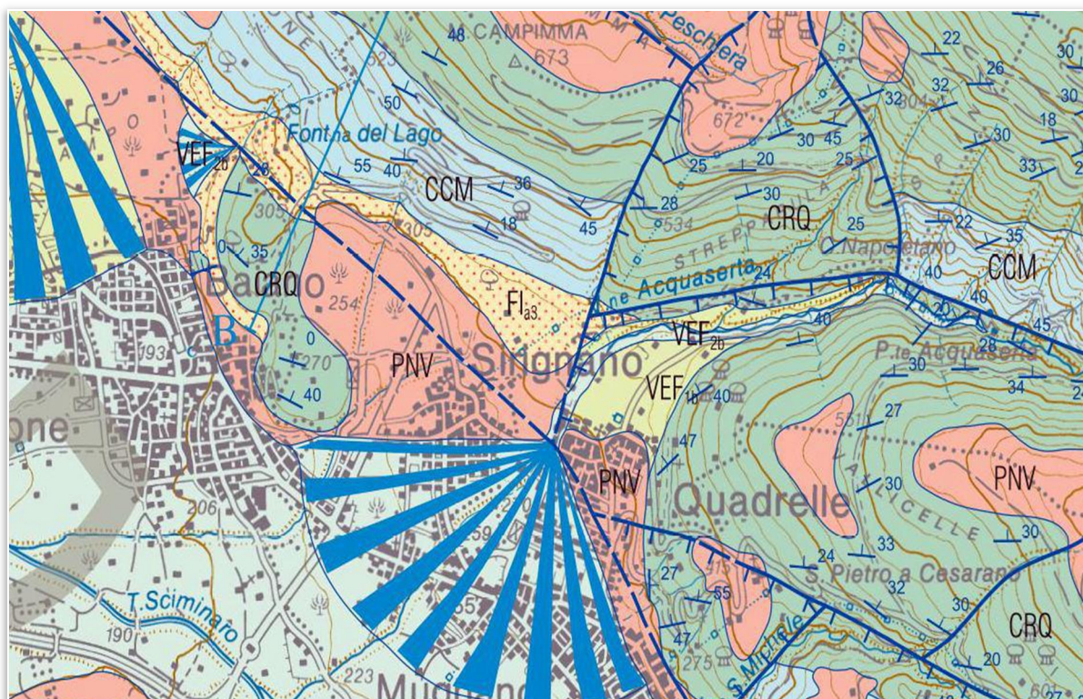
Figura 3 Stralcio Carta geologica d'Italia Foglio 488 "Ercolano" Scala 1: 50.000
