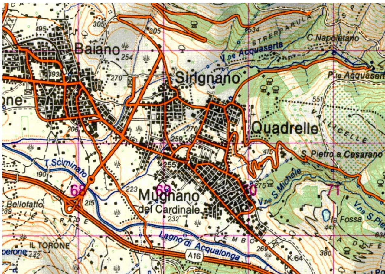
Figura 2 Stralcio Carta d'Italia, Foglio 448 "Ercolano" IGMI, scala 1:50.000
