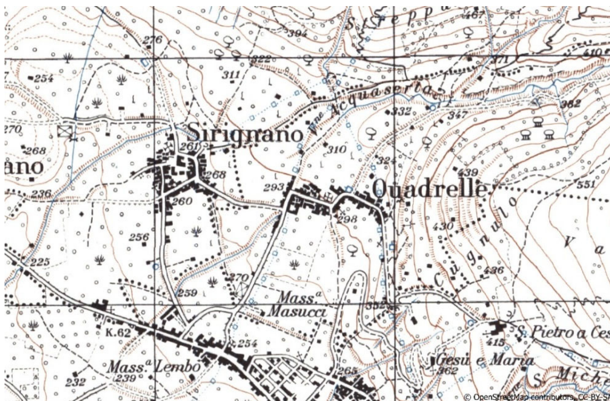
Figura 1 Stralcio IGM, Foglio IV NE “Baiano”, scala 1:25.000
