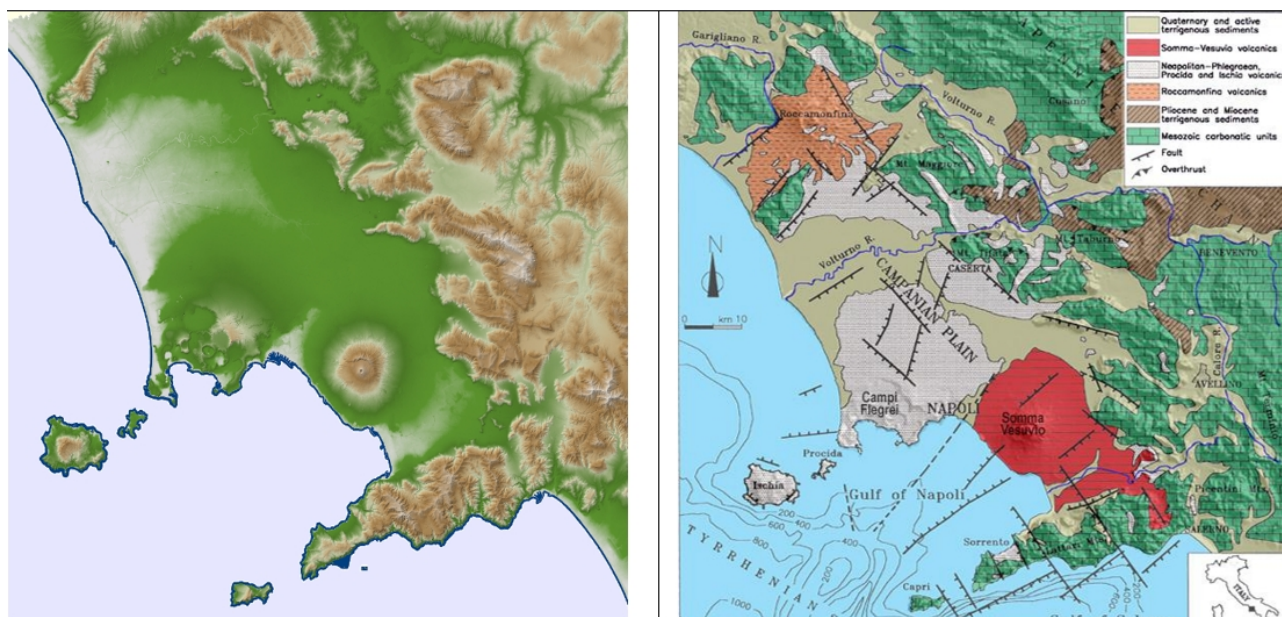
Figura 4 Immagine satellitare della dorsale appenninica e della piana campana e schema strutturale della Piana Campana e delle strutture bordiere
